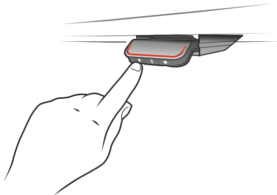
Abbildung 43: Favoritenpositionen löschen
