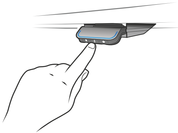
Abbildung 44: Bluetooth® verbinden
