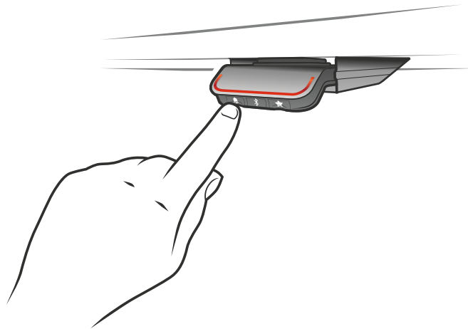
Abbildung 46: Erinnerung zurücksetzen
